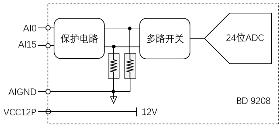
BD 9208 的电路示意图
